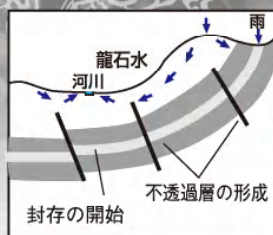
約1万年前の時の地殻変動
