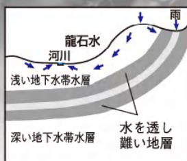
約1万年前以前の地下水状態 (封存水形成のイメージ図)
